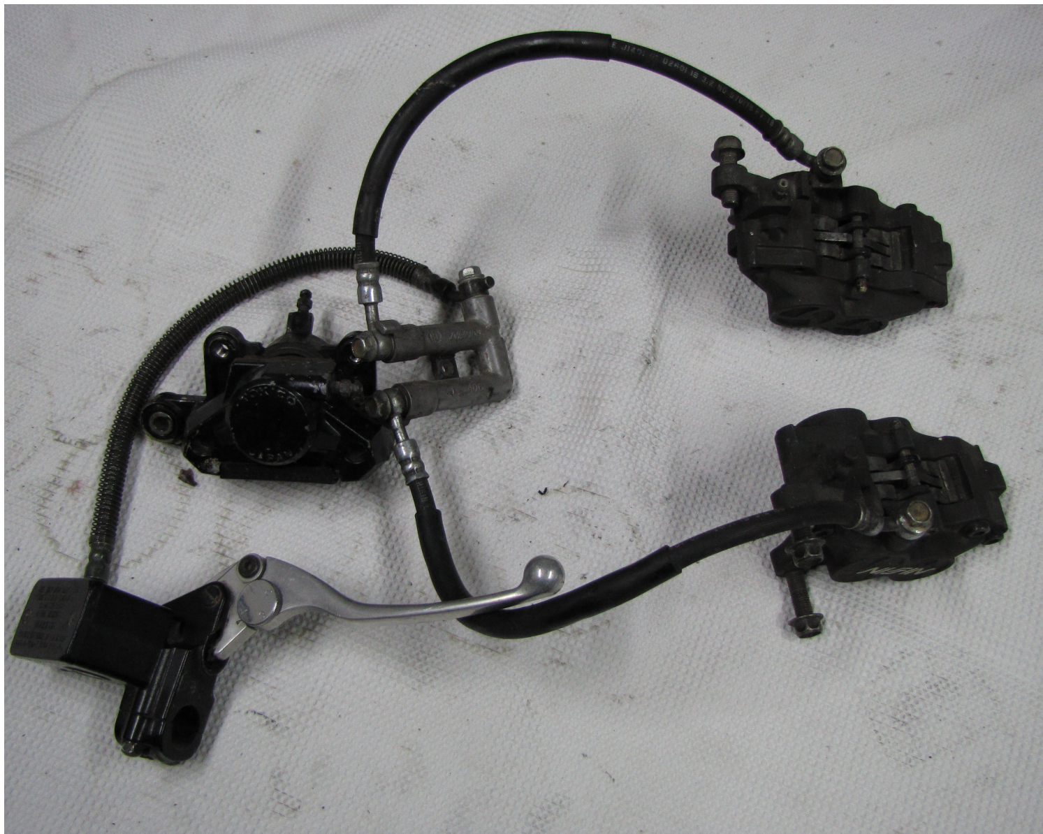
Impianto frenante pinze anteriori + pinza posteriore Suzuki GSXR
