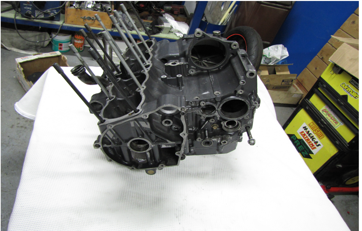
Carter motore completi Suzuki GSXR anno 1991 CC 1127
